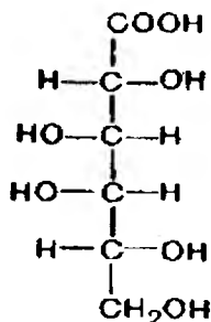
D-galakton kislota
