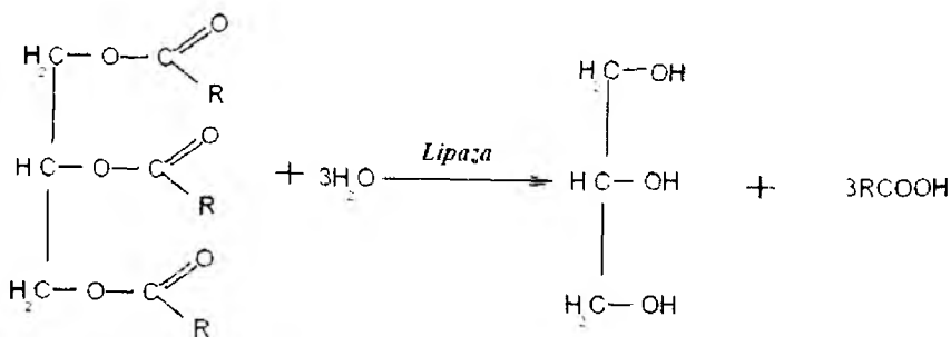
Triglitserot
