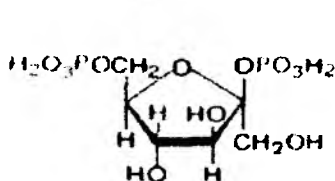
fruktoza-2,6-bifosfat
