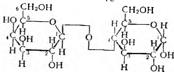
laktoza
