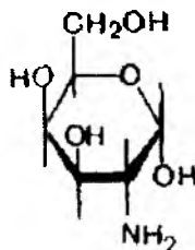
D-galakto-amin
