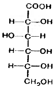
D-glyukon kislota
