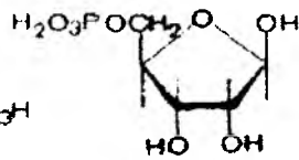
riboza-5-fosfat
