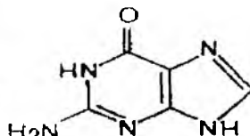
Guanin
