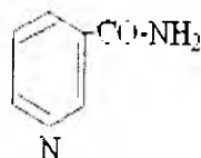
nikotinamid
