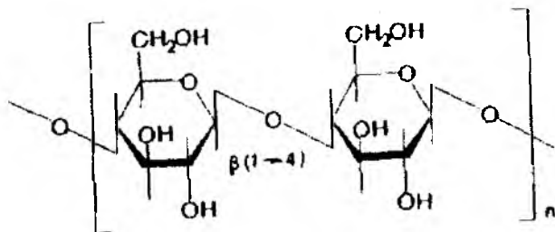
Sellyuloza molekulasi uchastkasi
