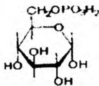
glyukoza-6-fosfat
