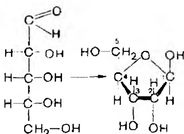
D- riboza
