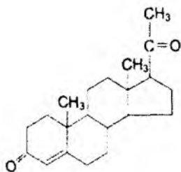
Progesteron
