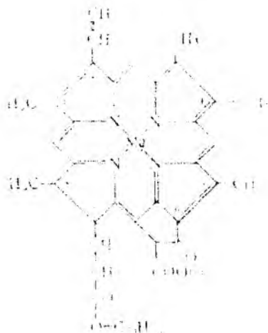
xlorofill a
