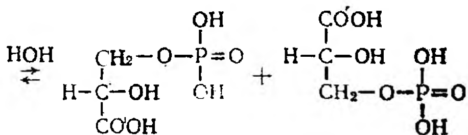
3-fosfoglitserrat kislota
