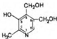
Piridoksin
