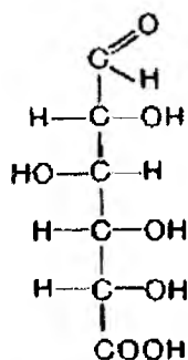
D-glyukouron kislota
