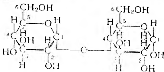
maltoza
