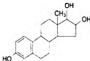
Esterol
