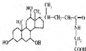
Glikoxolat kislota
