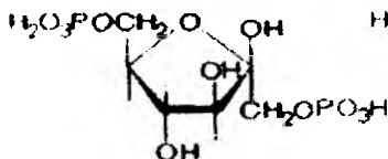
fruktoza-1,6-bifosfat
