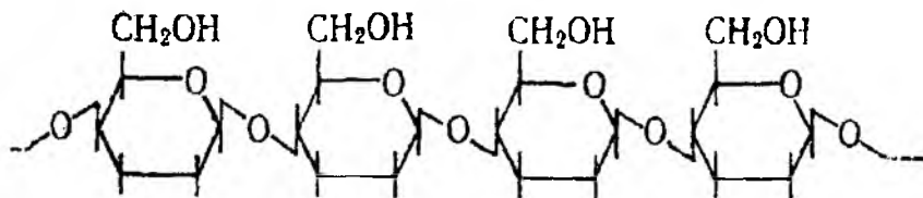
amiloza
