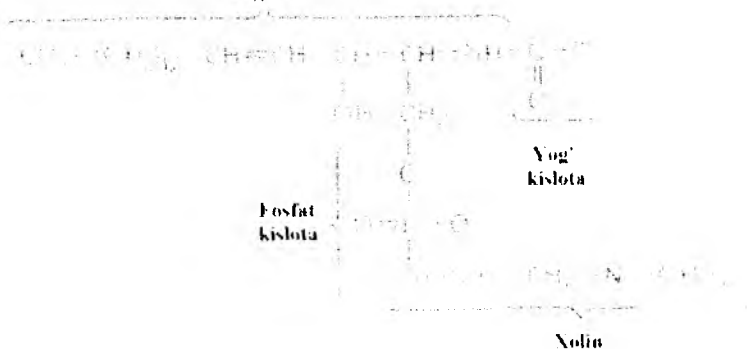
Sfingozin
