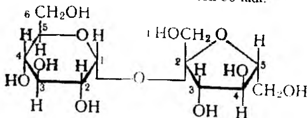
saxaroza
