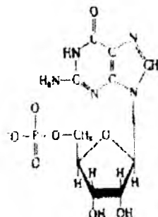
Guanilat, guanozin -5ʻ monofosfat (GMF)
