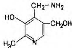
Pirididoksiamin
