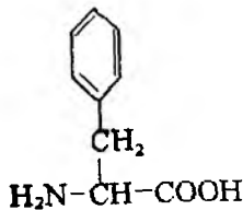
Fenilalanin
