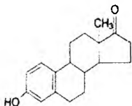
Esteron
