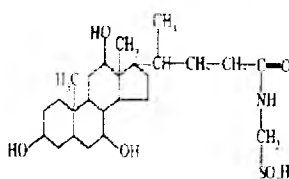
Tauroxolat kislota
