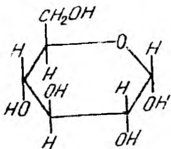
D - glyukopiranoza
