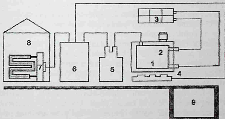
11.1-rasm. Biogaz va biogumus olish qurilmasining prinsipial sxemasi.
