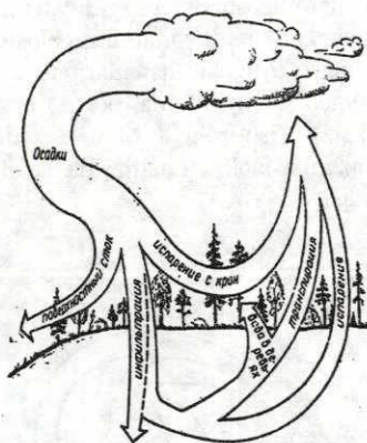
Круговорот воды в биосфере
