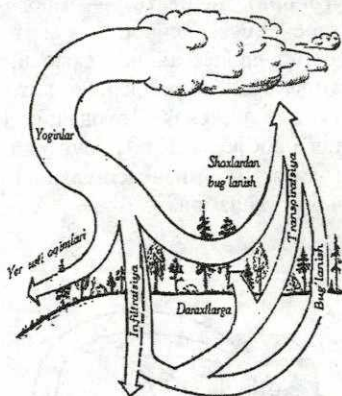
Suvning biosferada aylanishi
