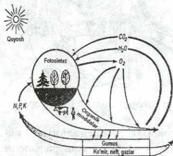
Эколизмларда биологик модда айланиши
