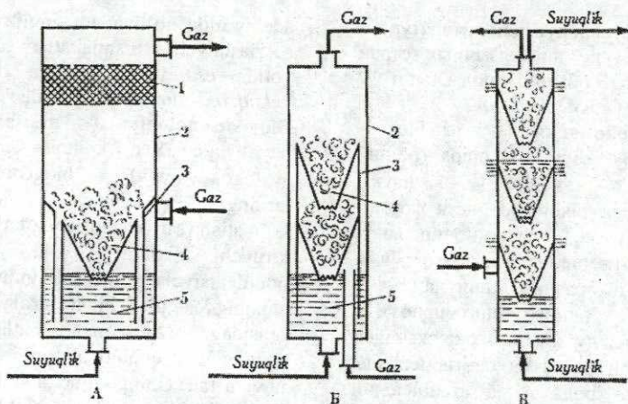
Конуссимон барботаж абсорберлари:
