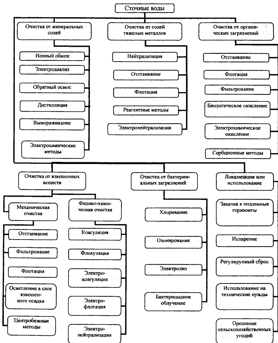
Классификация основных методов очистки и обеззараживания сточных вод на карьерах.
