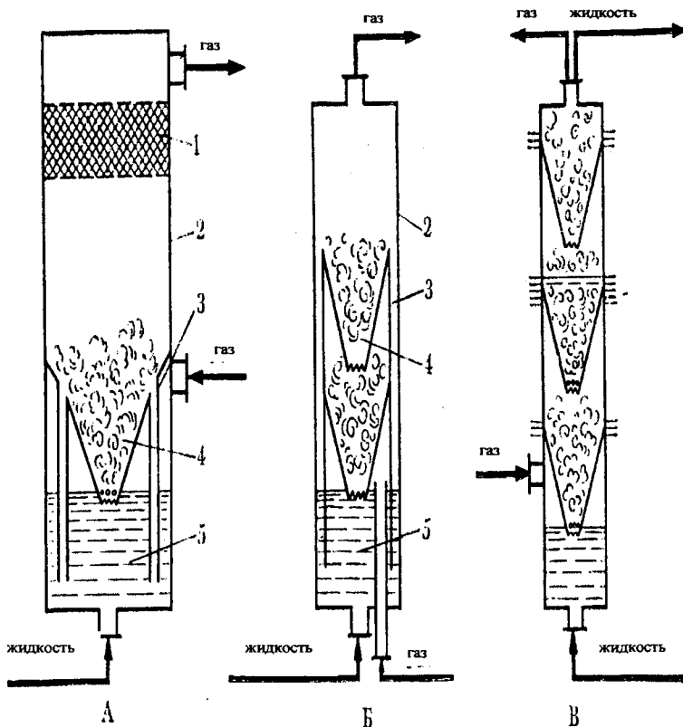
Конусные барботажные абсорберы. А,Б – абсорберы с периодической подачей жидкости, В – абсорбер с непрерывным прямотоком жидкости и газа: 1-брызгоотбойник, 2-корпус, 3-переточное устройство (трубки, зазор), 4-полный конус с отверстиями или пазами, 5-расходная ёмкость жидкости.
