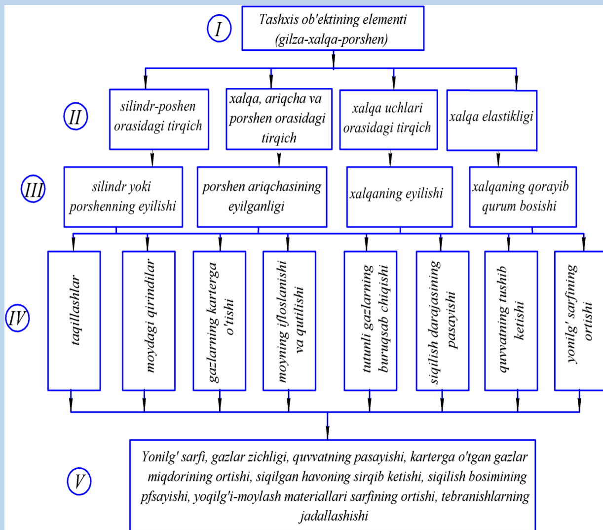
82-rasm. Tashxis ob'ekting strukturaviy modeli (dvigatelning silindr porshen guruxi misolida)
