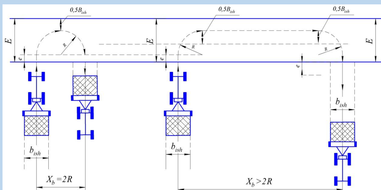
16-rasm. Sirtmoqsiz burilish joyida agregatlarning parakatlanish troektoriyasi
